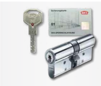
ES 2200 BKS Janus Profilzylinder mit Sicherheitskarte gemäß DIN EN 1303 und DIN 18252 Wendeschlüsseln
